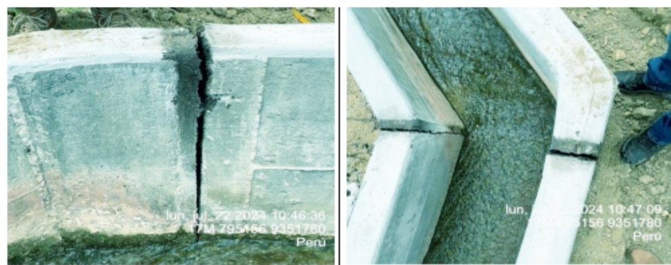
Se visualiza separación de muros de concreto de canal y juntas que carcon inadecuado relleno o sello asfáltico.
